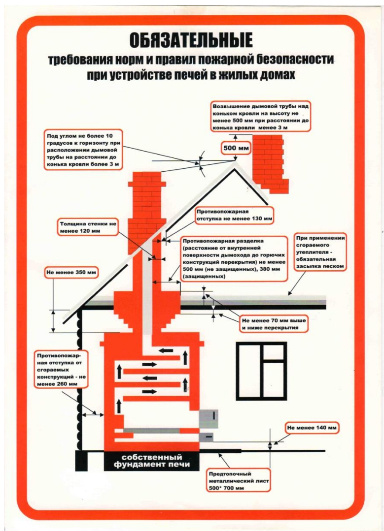
Рисунок 35. Обязательные требования норм и правил пожарной безопасности при устройстве печей в жилых домах
